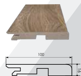
Плинтус
