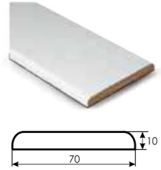
Наличник плоский
