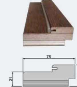
Стойка коробка скрытая алюминиевая внутреннего открывания
