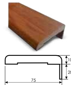
Наличник телескопический
