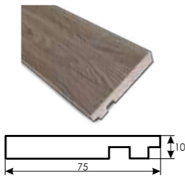
Наличник копланарный
