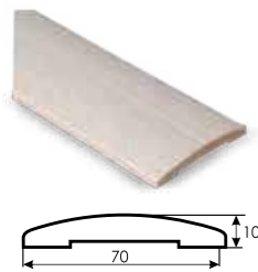
Наличник полукруглый
